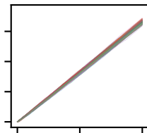
AEG
